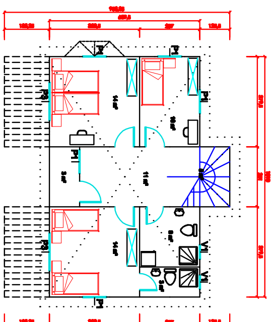
66 m 2 PREFABRIKE BINA 1. KAT PLANI
