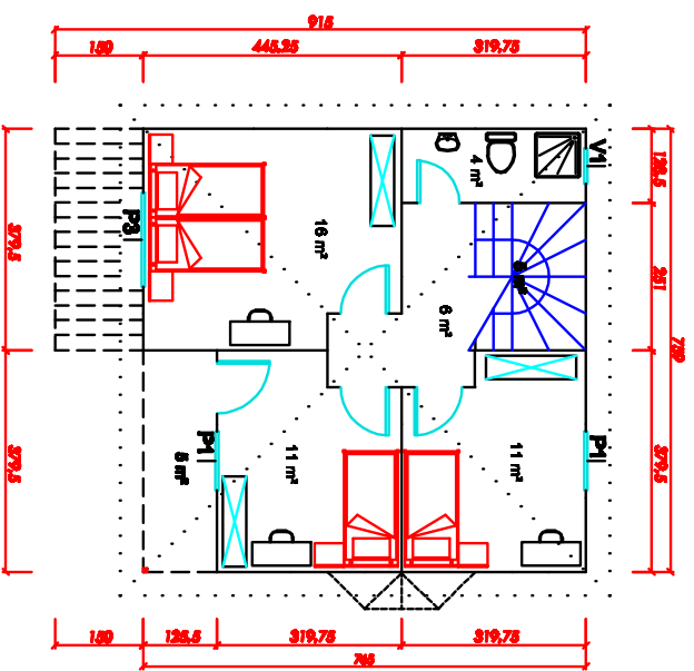
58 m 2 PREFABRIKE BINA 1. KAT PLANI
