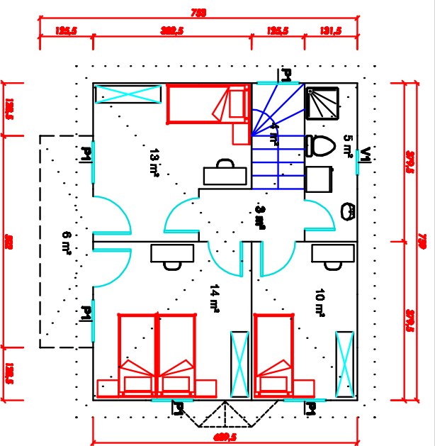
55 m 2 PREFABRIKE BINA 1. KAT PLANI
