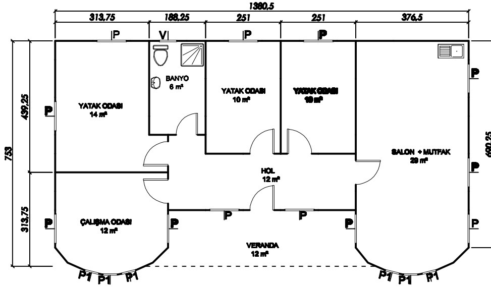
105m² PREFABRİK KONUT BİNA PLANI ( 93 m² + 12 m² veranda = 104 m² )
